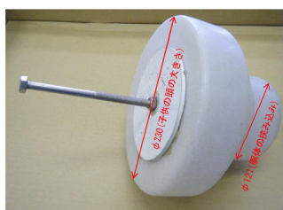
写真2-JPFA 点検器具 A （通り抜ける寸法）
